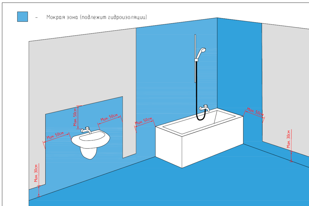
Рис. 35.2 Мокрые зоны внутри влажных помещений, подлежащие гидроизоляции.
