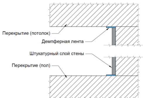
Рис.28. Приклейка демпферной ленты в местах сопряжения штукатурного слоя со стеной и потолком
