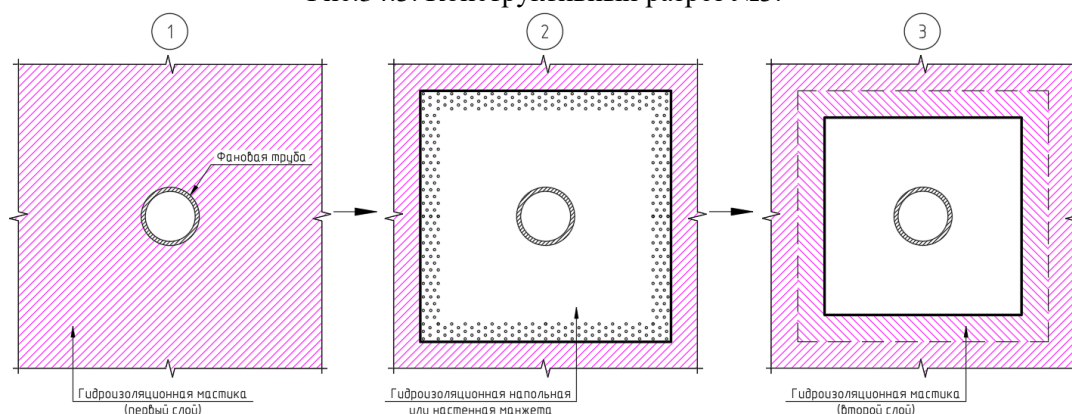
Рис.34.4. Последовательность нанесения гидроизоляционной манжеты
