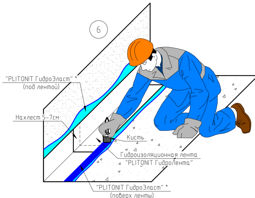
Рис.35.1. Последовательность работ (на стенах работа в аналогичном порядке), где: 1 - проверка ровности основания контрольной рейкой (аналогично для горизонтальной поверхности); 2 – размешивание емкости с мастикой; 3 – нанесение первого слоя мастики, разбавленной водой в пропорции 1:10, на основание; 4 – нанесение гидроизоляции на поверхность (аналогично для горизонтальной поверхности); 5 – укладка гидроизоляционной ленты на поверхность, предварительно обработанную «PLITONIT ГидроЭласт» или «PLITONIT WaterProof Standard»; 6 – поверхностная обработка ленты мастикой «PLITONIT ГидроЭласт» или «PLITONIT WaterProof Standard».
