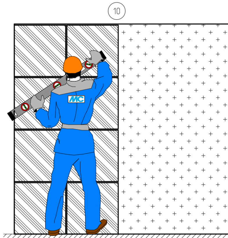
Рис.37. Последовательность работ, где: 1 – проверка ровности основания контрольной рейкой; 2, 3 – приготовление грунтовки; 4 – нанесение грунтовки на цементную штукатурку; 5 – приготовление клеевой смеси; 6, 7 – нанесение клеевой смеси на основание (захватками); 8, 9 – приклеивание керамогранитной плитки на стену (захватками); 10 – проверка облицовки при помощи уровня. ПРИМЕЧАНИЕ к рис 37.: на этапах 6-9 указано проведение работ в направлении снизу вверх, но при использовании клеев, в маркировке которых присутствует буква «Т», возможно выполнение работ в направлении сверху вниз.
